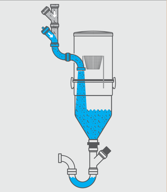
1ª FASE AO INICIAR A ASPIRAÇÃO, A ELECTROVÁLVULA ACCIONA O INJECTOR DE ÁGUA QUE SE IRÁ MISTURAR COM O PÓ ASPIRADO.
