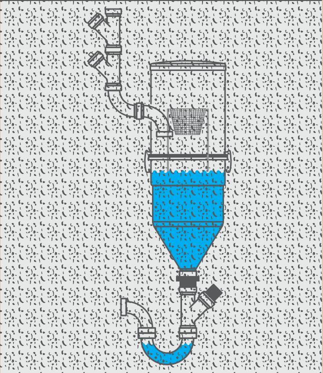
2ª FASE ASSIM QUE A ÁGUA CHEGA AO NÍVEL DOS SENSORES, A ASPIRAÇÃO PARA E A ENTRADA DE ÁGUA É INTERROMPIDA.
