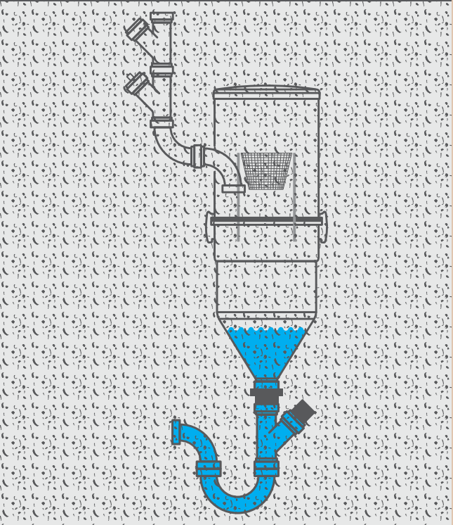
3ª FASE ABRE-SE A VÁLVULA DE DESCARGA E É FEITA A DESCARGA PARA O ESGOTO, VOLTANDO À PRIMEIRA FASE.
